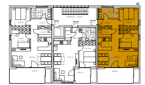
2 Obergeschoss HAUS A
