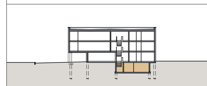
SCHNITT
